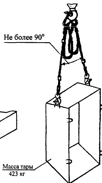
Строп 4СК1-5,0÷4СК1-10,0 Q = 5 \div 10 тс при выгрузке ящика
