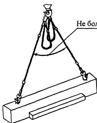
Строп 4СК1-3,2 4СК1-5,0 4СК1-10,0 Q = 3,2 \div 10,0 тс (2СК-5,0) при монтаже ригелей P = 0,3 \div 4,4 т
