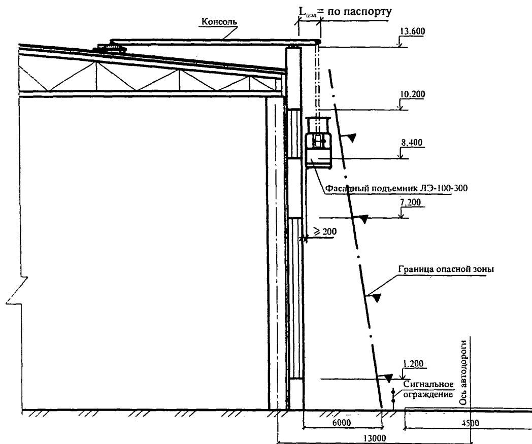
Рис. 38. Схема привязки фасадного подъемника для устройства остекления
