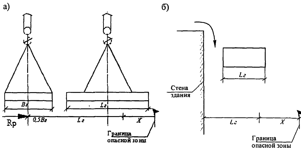
Рис. 13. Границы зон при работе стрелового крана (крана-манипулятора)
