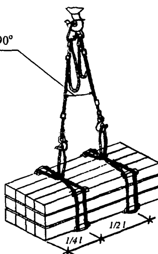
Строп 4СК1-3,2÷4СК1-10,0 Q = 3,2÷10,0 тс при подаче пиломатериалов V = 2 м³ Р = 1,6 т
