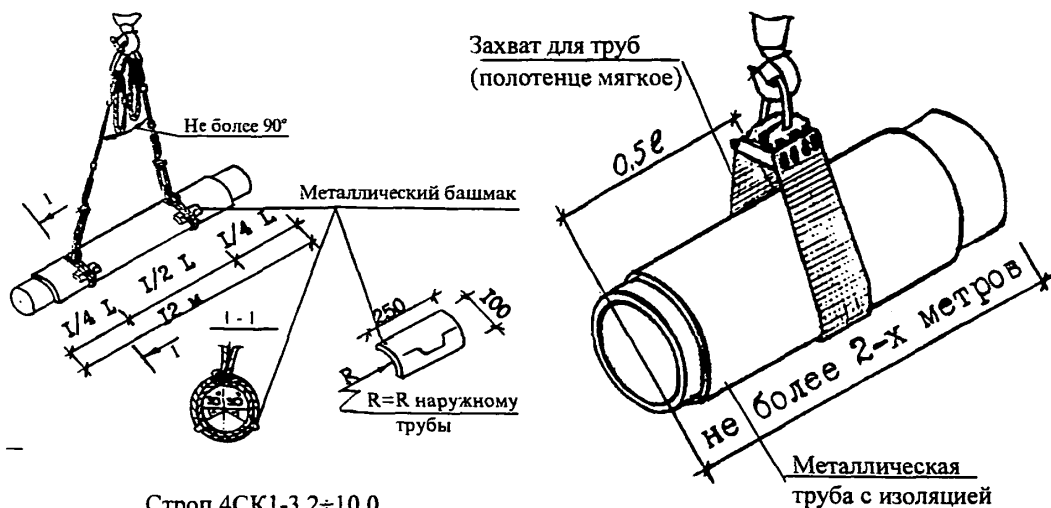
Строп 4СК1-3,2÷10,0 Q=3,2÷10,0 тс при подаче трубы с гидроизоляцией \varnothing 50÷100 мм P до 1,0 т
