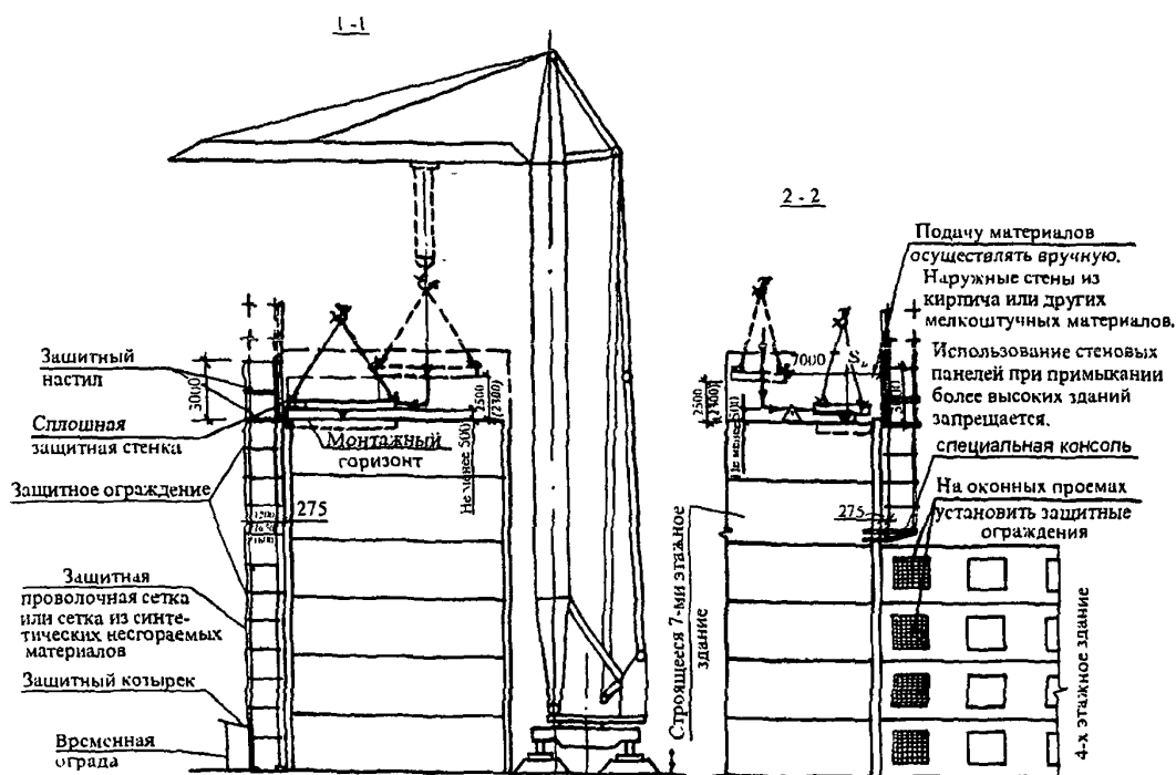
Рис. 24. Разрезы 1-1 и 2-2
