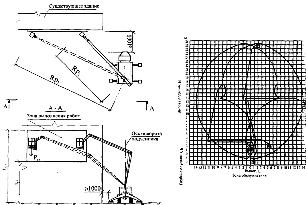
Рис. 7. Привязка подъемника (вышки)
