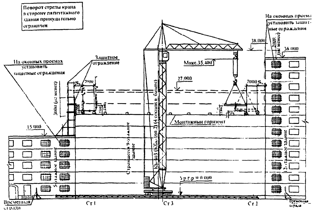
Рис. 22. Разрез 1-1
