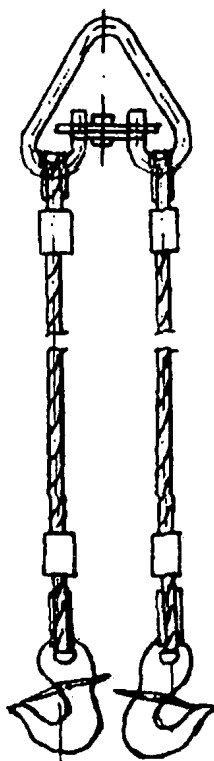
Строп канатный двухветевой типа 2СК ГОСТ 25573-82*
