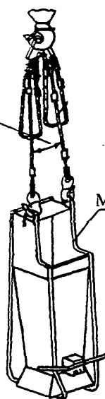
Строп 4СК1-10,0 Q = 10,0 тс при подаче бункера (бадьи) с бетонной смесью V = 1,0 \text{ м}^3 P = 3,0 т
