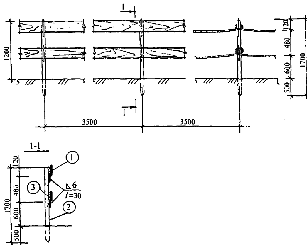
Рис. 31. Временное ограждение рельсовых крановых путей (вариант 2)
