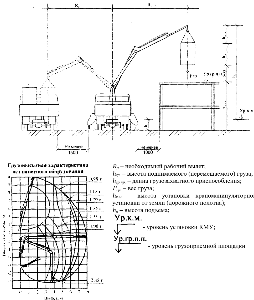
Рис. 5. Привязка крана-манипулятора
