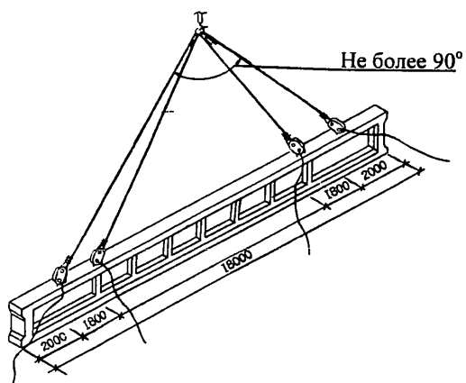
Строп 2СК-10,0
