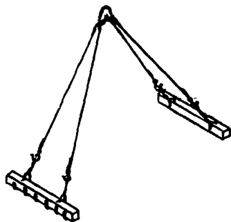
Траверса для подъема карт из профнастила
