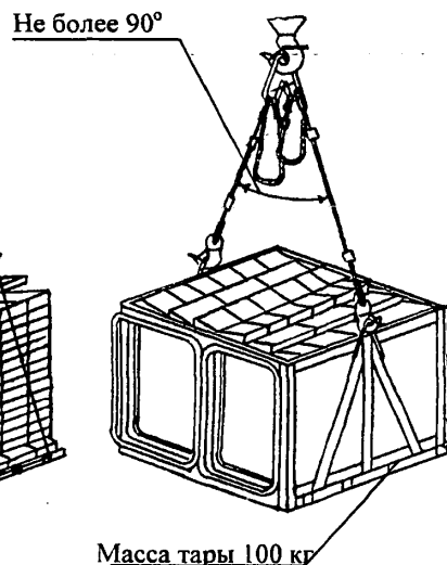
Строп 4СК1-5,0÷4СК1-10,0 Q = 5,0÷10,0 тс при разгрузке с автотранспорта кирпича в траверсном футляре Р = 1,7 т
