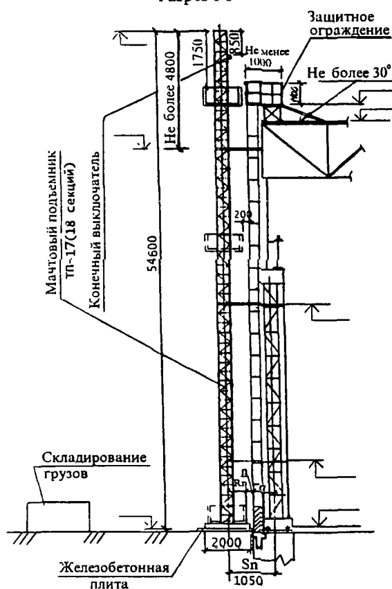
Разрез I-I
