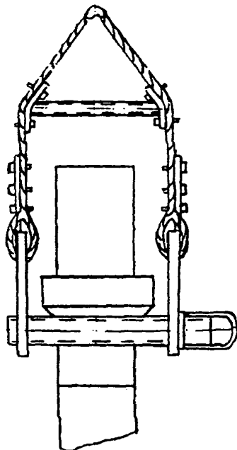
Строп канатный кольцевой типа СКК1 ГОСТ 25573-82*
