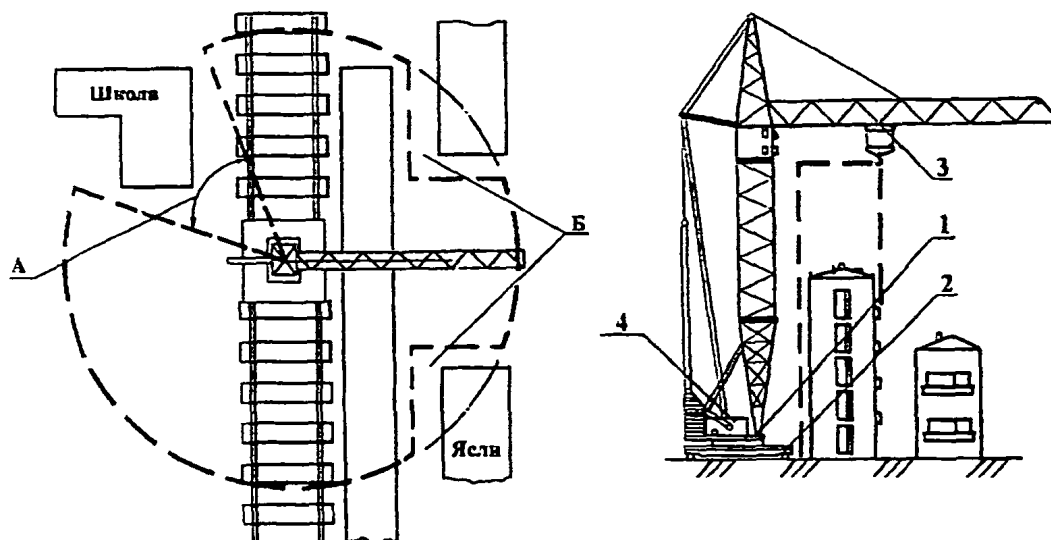
А – ограничение поворота стрелы; Б – ограничение вылета грузовой тележки. 1 – датчик ограничения угла поворота; 2 – датчик ограничения перемещения крана; 3 – датчик ограничения изменения вылета; 4 – датчик ограничения высоты подъема крюка Рис. 26. Схема действия системы ограничения зон работы СОЗР башенного крана
