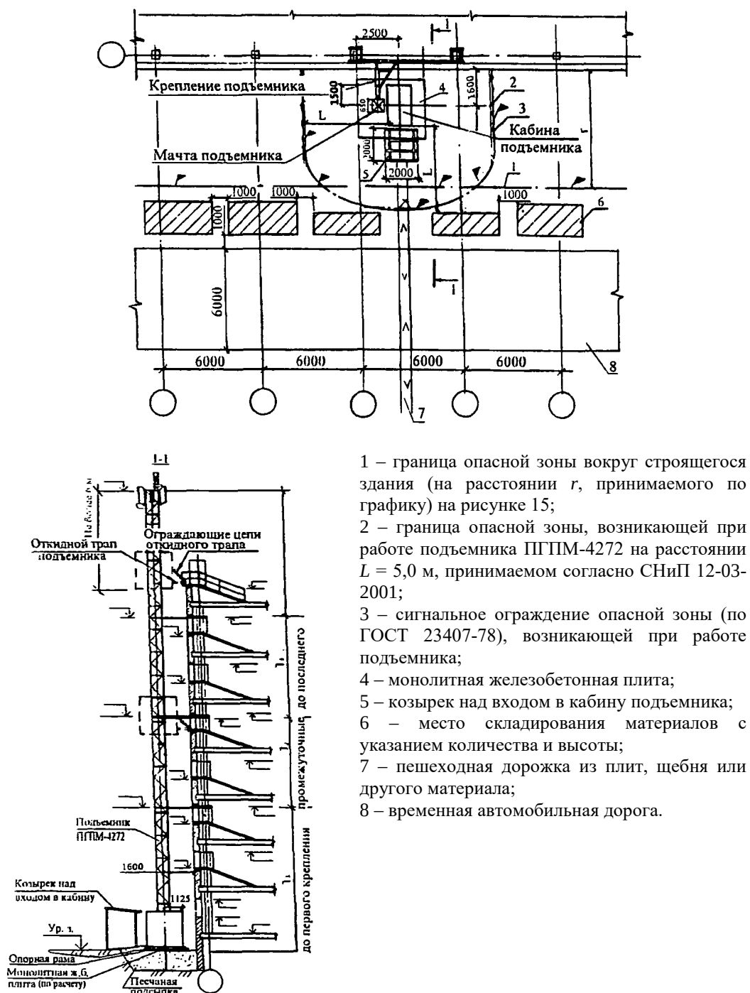
Рис. 36. Установка пассажирского подъемника ПГПИМ-4272 у здания
