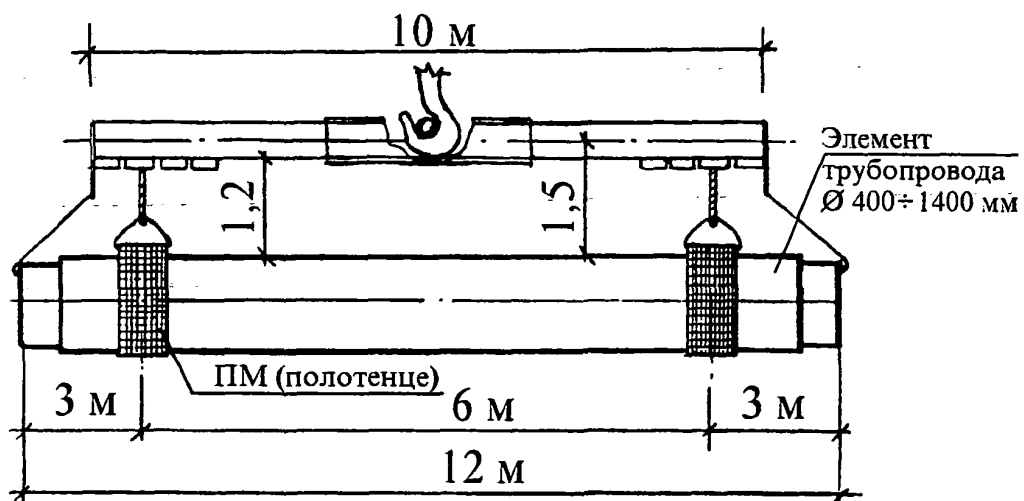
Траверса для разгрузки труб \varnothing 400÷1400 мм Q=18 тс, P=1530 кг
