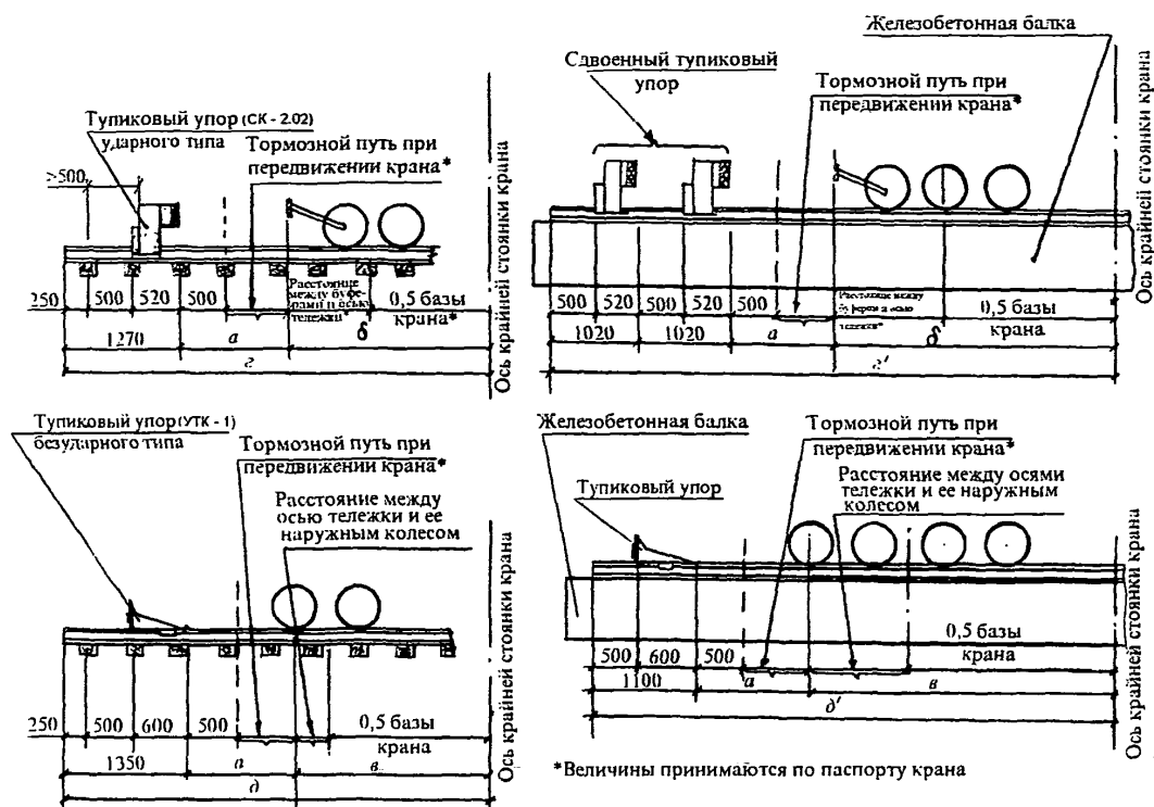
Рис. 40. Привязка тупиковых упоров и крайних стоянок кранов к концам рельсового пути
