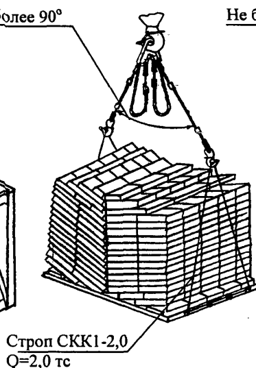
Строп 4СК1-3,2÷4СК1-10,0 Q = 3,2÷10,0 тс при разгрузке с автотранспорта кирпича на поддонах Р = 1,6 т
