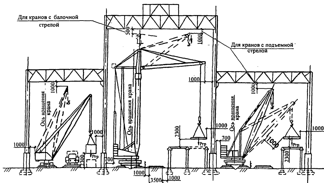
Рис. 11. Привязка крана внутри строящегося или реконструируемого здания
