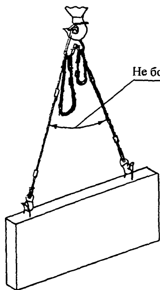
Строп 4СК1-3,2 4СК1-5,0- 4СК1-10,0- (2СК-5,0) (2СК-5,0) Q=5,0 \div 10,0 тс Q=3,2 \div 10,0 тс Q=5,0 \div 10,0 тс при монтаже стеновых панелей P = 0,71 \div 2,45 т
