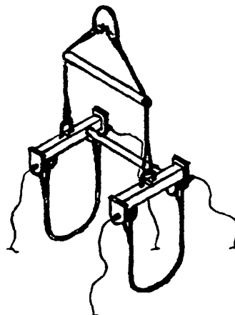
Траверса для подъема двухветвевых железобетонных колонн
