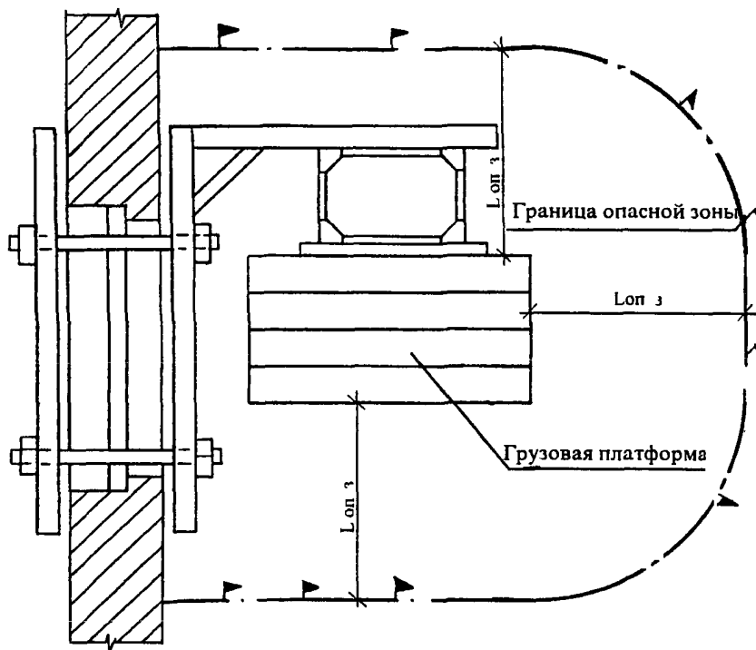
Рис. 16. Опасная зона при работе грузового строительного подъемника
