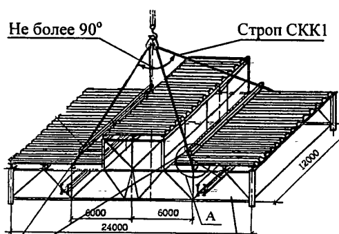
Блок покрытия пром.зданий P_{max}=22 т
