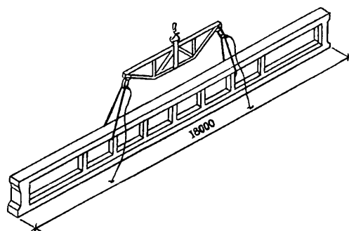
Траверса TP20-5
