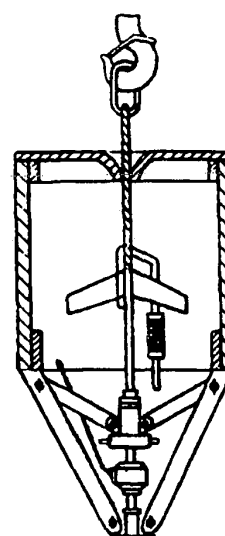
Грузозахватное приспособление для монтажа ствола мусоропровода
