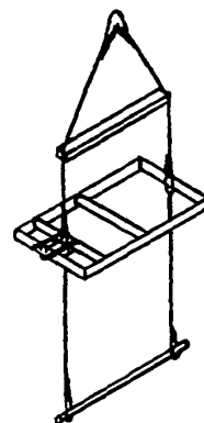
Траверса для подъема металлических двухветвевых колонн
