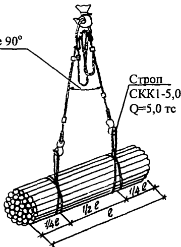
Строп 4СК1-3,2÷4СК1-10,0 Q = 3,2 \div 10,0 тс при подаче арматурных стержней P = 1,0 т
