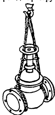
Стропы СКК1-1,6 и СКК1-5,0 Q = 1,6÷5,0 тс при монтаже задвижки \varnothing 150÷600 мм P = 0,2÷3,0 т
